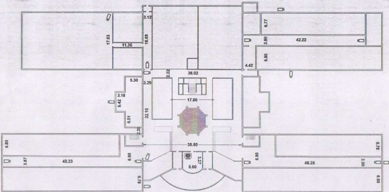
План 1 этажа
